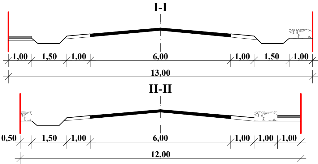
ПОПЕРЕЧНІ ПРОФІЛІ I-I; II-II М 1:100
